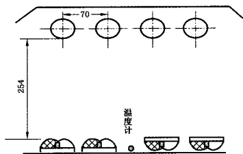
图 A.2 紫外线曝晒形式
